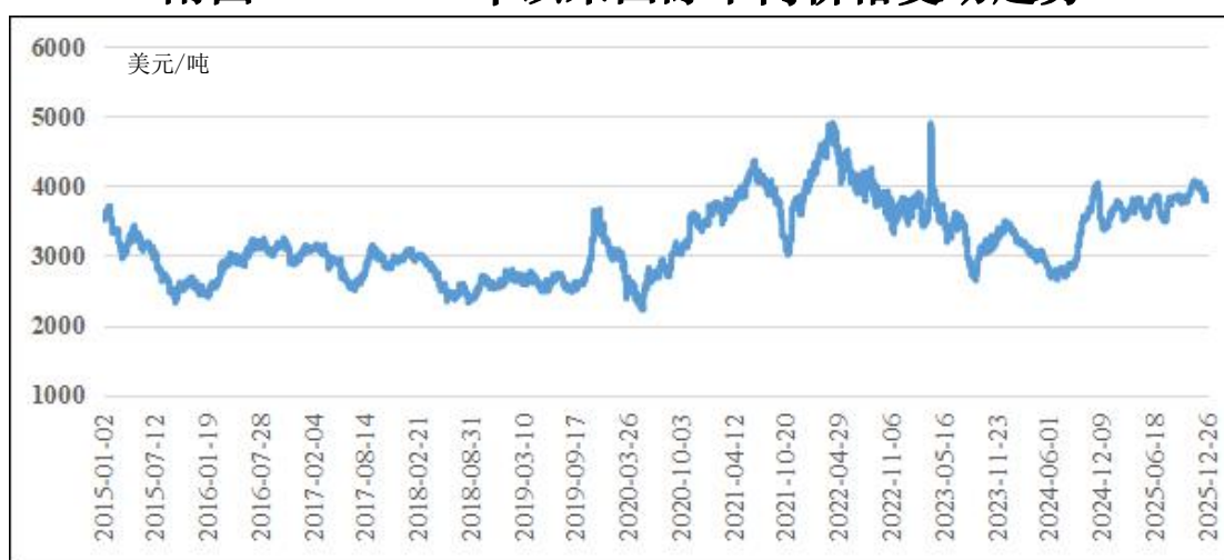
附图 11 2015 年以来 FAO 食品价格指数变动趋势
